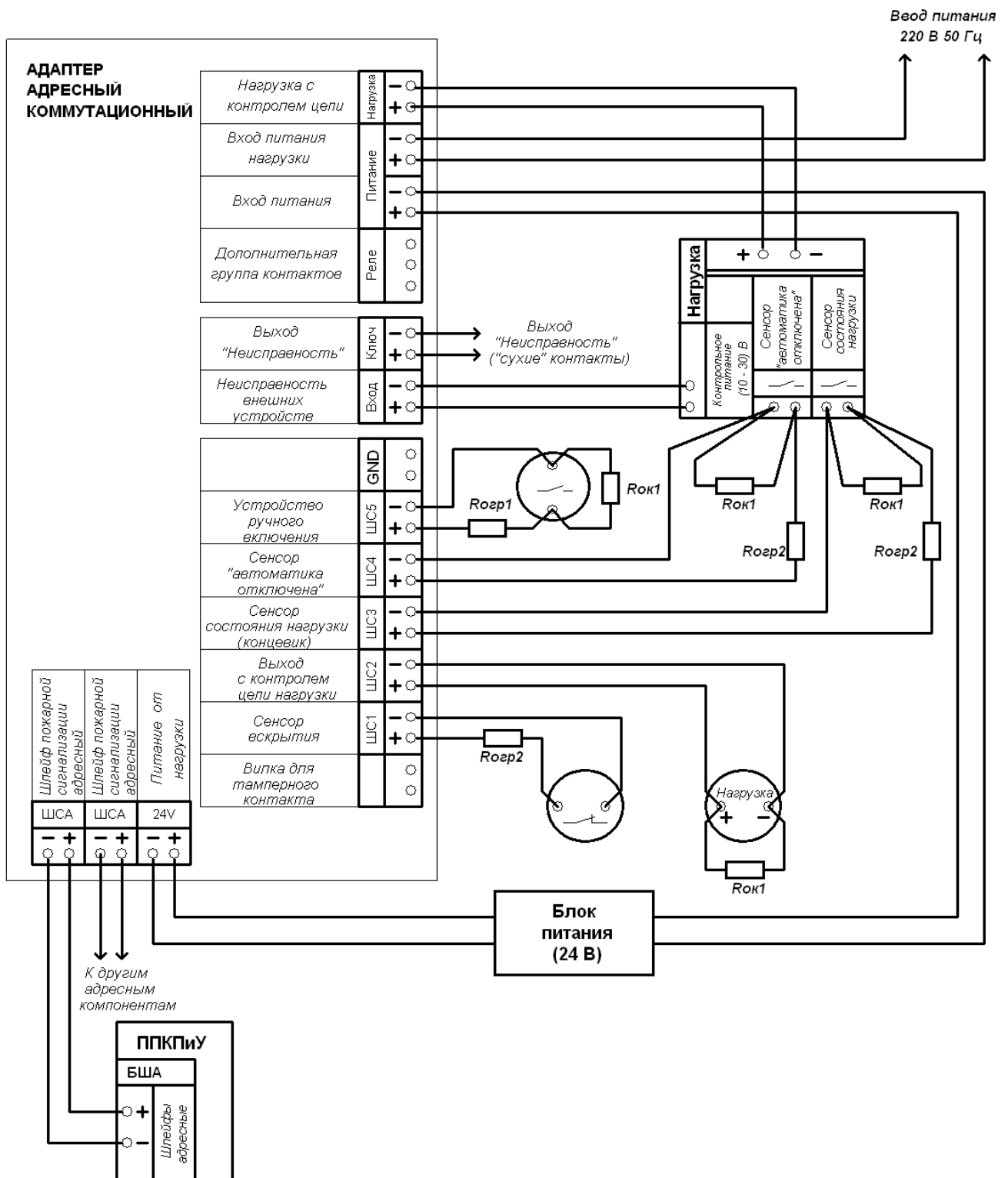
Рисунок П20.12 - Схема подключения ААК (вариант исполнения питания нагрузки 220 В 50 Гц)
