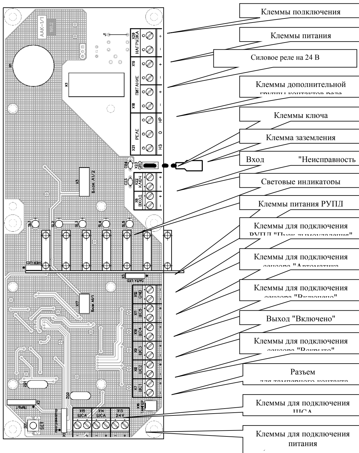
а) вариант исполнения с питанием 24 В постоянного тока и релейным выходом
