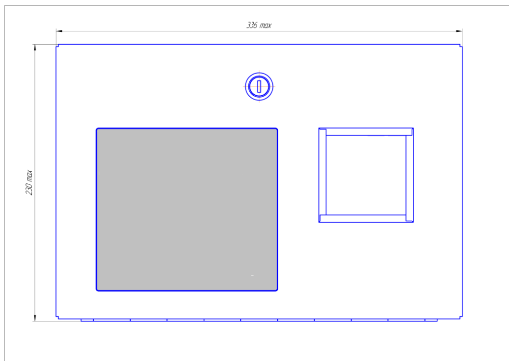
Рис. ПЗ.12. Вариант исполнения 1
