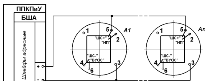
Рисунок П20.6 - Схема подключения адресных пожарных извещателей (ИПА).
