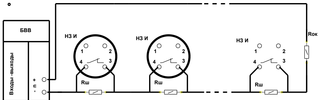
Рисунок П20.3 - Схема подключения извещателей, выключателей и кнопок управления (пассивных, работающих на уменьшение тока в ШС и имеющих НЗ контакт)
