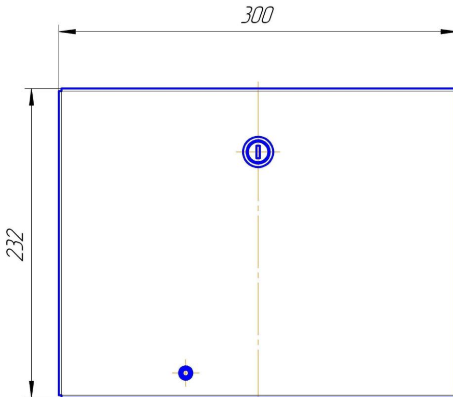
Рис. ПЗ.14. Вариант исполнения 1
