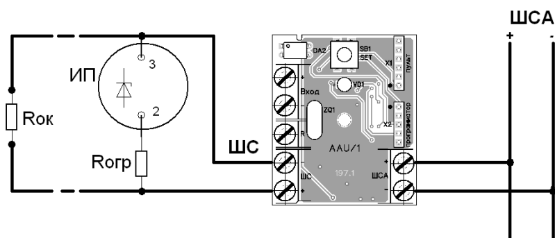
Рисунок П20.8 - Схема подключения извещателей (активных, работающих на увеличение тока в ШС и имеющих падение напряжения от 5 В до 8 В в режиме "Тревога") к ААУ.
