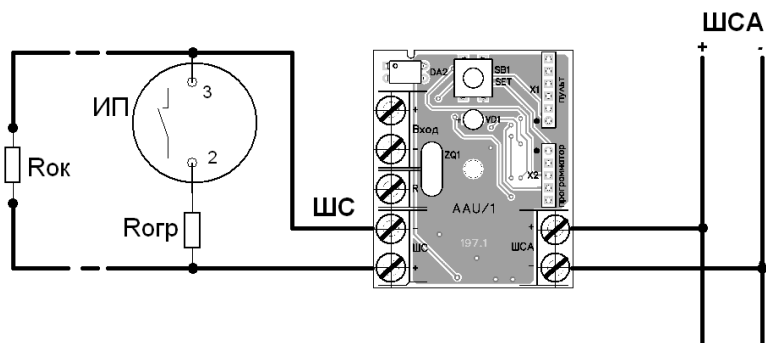
Рисунок П20.9 - Схема подключения извещателей, выключателей и кнопок управления (активных, работающих на увеличение тока в ШС и имеющих НР контакт) к ААУ
