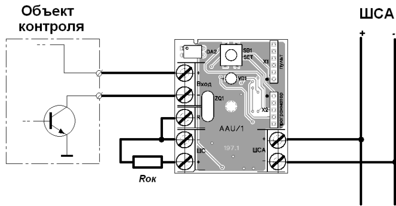
Рисунок П20.10 - Схема подключения ААУ к объекту контроля и ШСА.
