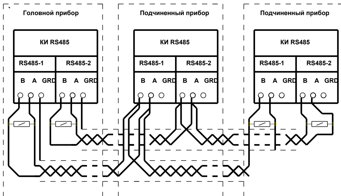
Рисунок П20.13 - Рекомендуемые схемы подключения приборов группы с применением КИ RS485.
