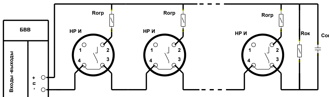
Рисунок П20.2 - Схема подключения извещателей, выключателей и кнопок управления (активных, работающих на увеличение тока в ШС и имеющих НР контакт)
