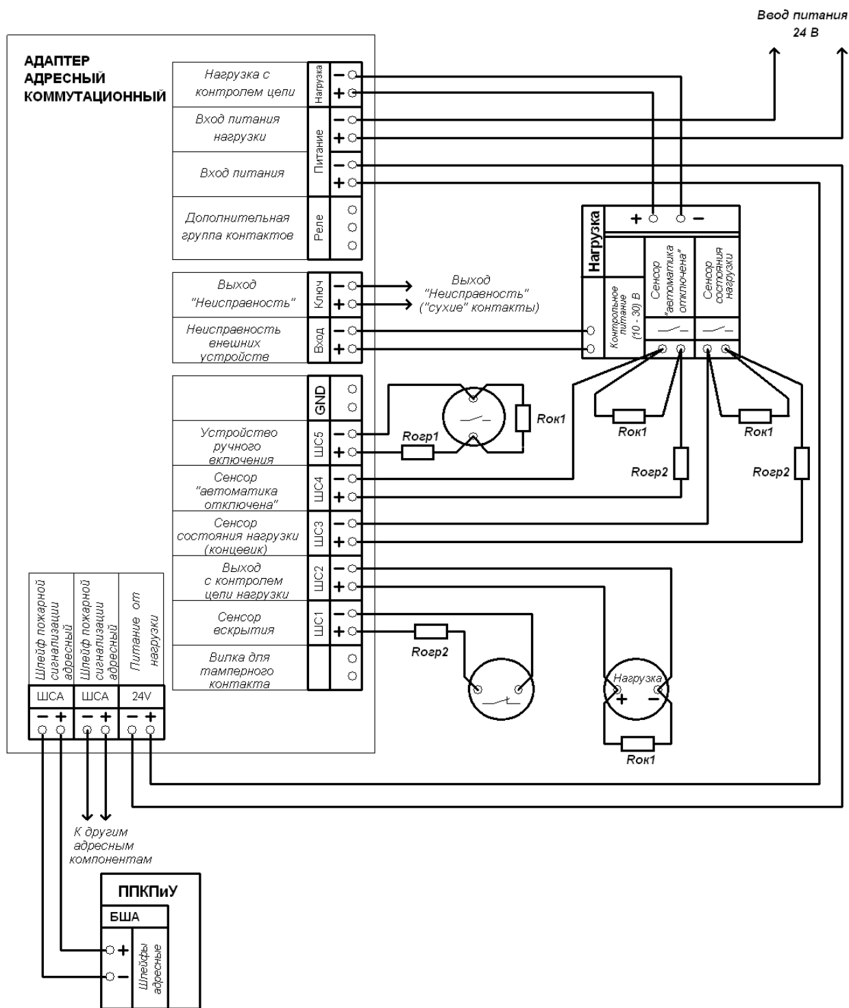
Рисунок П20.11 - Схема подключения ААК (вариант исполнения питания нагрузки-24 В)
