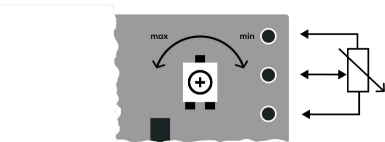
Рис.3 Підключення зовнішнього регулятора
