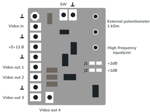
Рис.2 Розташування контактів
