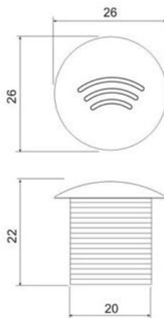
Зчитувач Mifare
