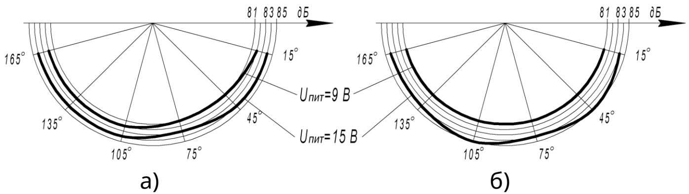
Рисунок 1 – Акустичні діаграми оповіщувача: а) – робоче положення, б) – повернене на 90 о за годинниковою стрілкою положення
