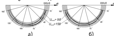
Рисунок 1.1 – Акустичні діаграми ОСЗ Джміль-1:
