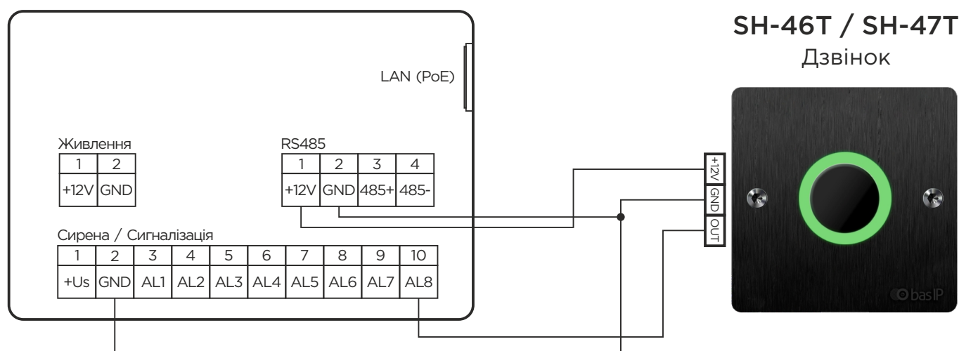
Схема підключення кнопки як дверного дзвінка
