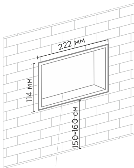
Монтажна коробка
