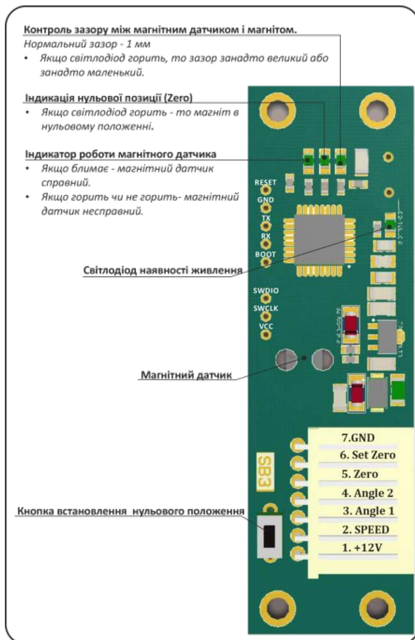
Рис. 23 – Опис контролера магнітного датчика
