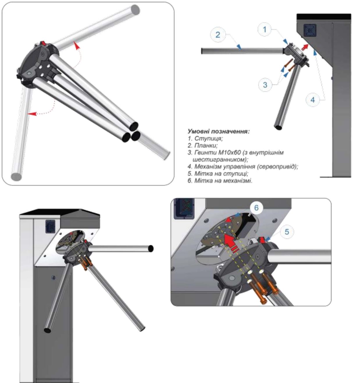
Рис. 15 – Встановлення ступиці з планками в корпус турнікету-триподу
