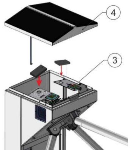
Рис. 20 – Встановлення зчитувача в турнікет-трипод
