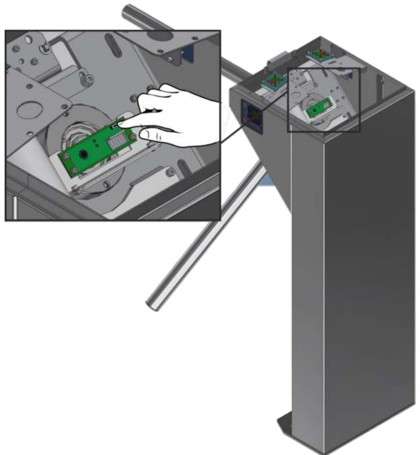
Рис. 21– Встановлення нульового положення ступиці
