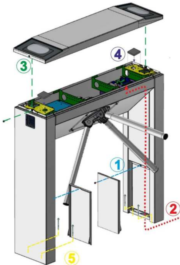
Рис. 17 – Загальний вид складання турнікету-триподу «TWIX-M»
