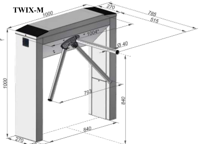
Рис. 3 -Габаритні розміри турнікета-трипода
