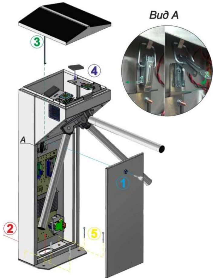
Рис. 16 – Загальний вид складання турнікету-триподу «CENTURION-M» і «BASTION-M»
