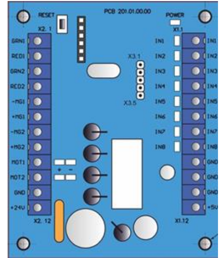
Рис. 10 – Зовнішній вигляд контролера моторизованого механізму РСВ.201.01.00.00
