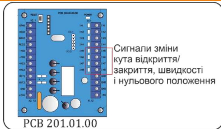
Рис. 22 –Сигнали зміни кута повороту на контролері PCB 201
