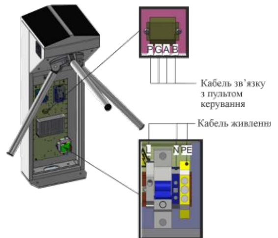
Рис. 19 – Підключення кабелю живлення і кабелю зв'язку з пультом керування
