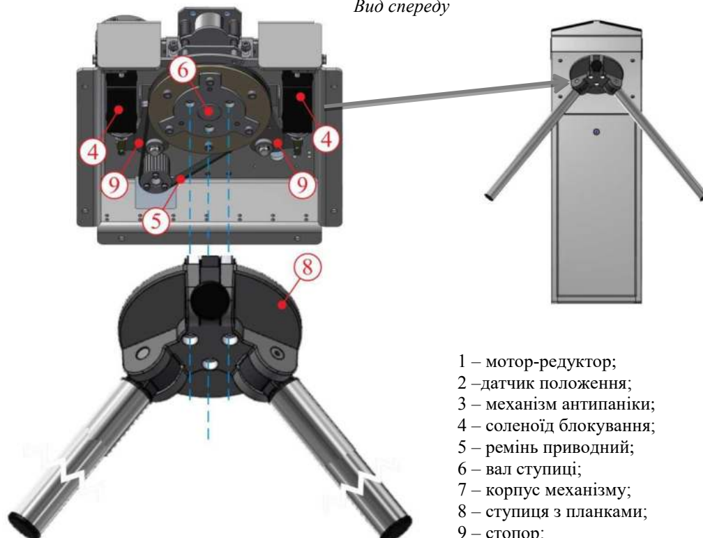
Рис. 5 – Робочий механізм турнікету
