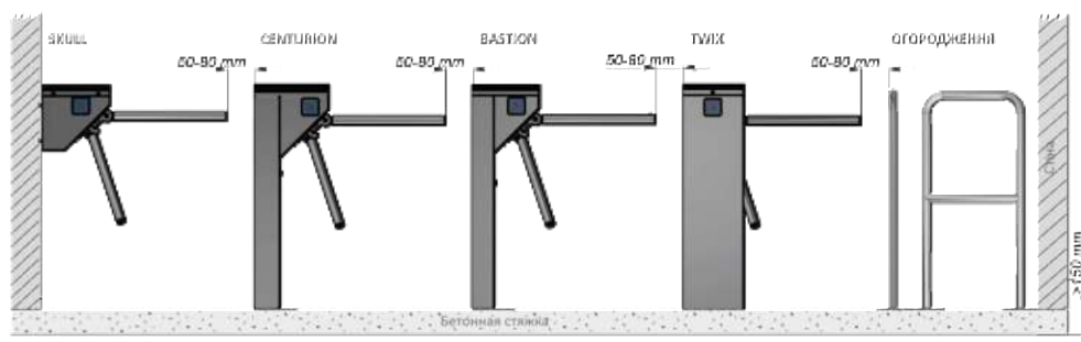
Рис. 12– Варіанти розміщення турнікетів-триподів (умовно)
