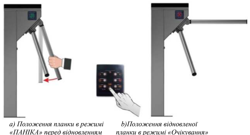
Рис.8 – Деактивація режиму «ПАНІКА» і відновлення планки у вихідне положення
