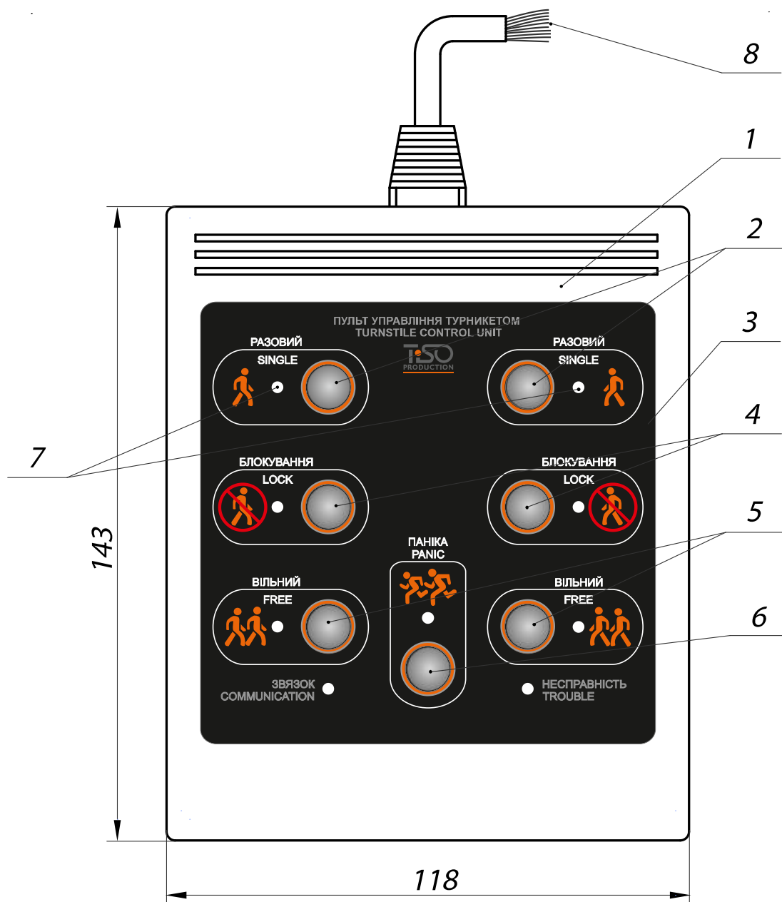
Додаток Б. Пульт управління та схема підключення
