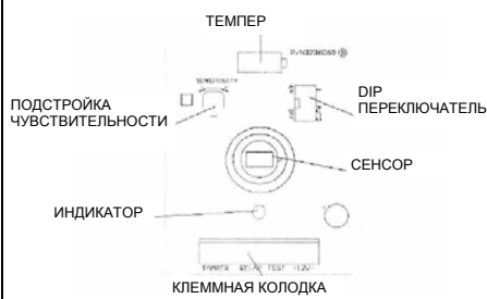
Рис. 3. LC-360. Вид платы
