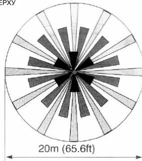
Рис. 5. LC-360. Схема зоны обнаружения
