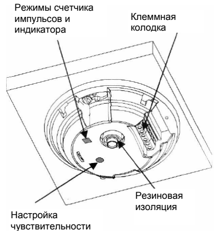
Рис. 2. LC-360. Вид без крышки
