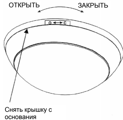
Рис. 1. LC-360. Вид корпуса
