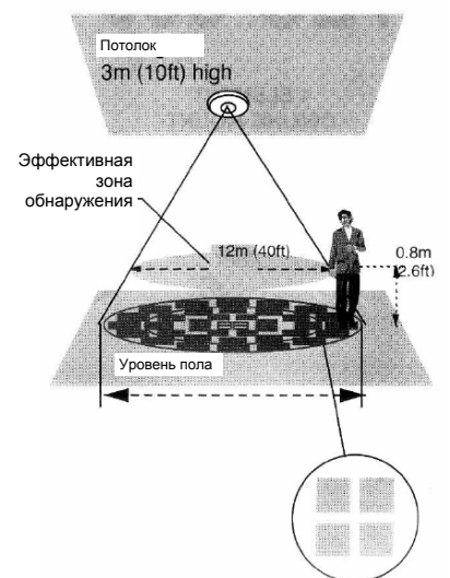
Рис. 4. LC-360. Зона обнаружения
