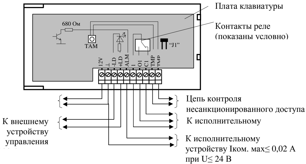
Рисунок Б.1 - Пример подключения клавиатуры Дунай-КА
