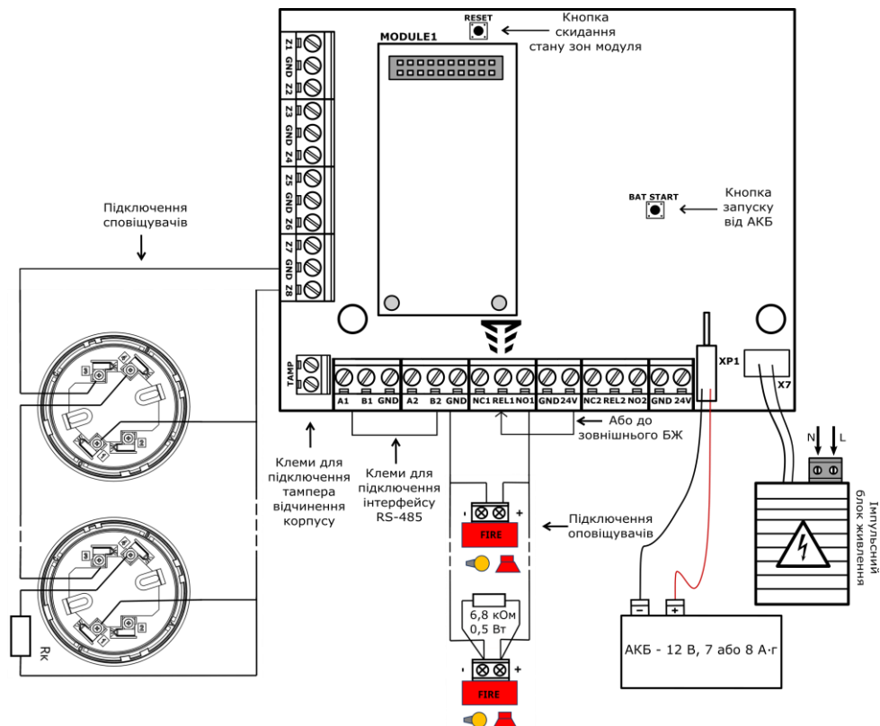
Рисунок А.1 – Зовнішній вигляд плати модуля M-ZP fBox
