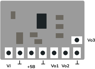
Рис.2 Розташування контактів
