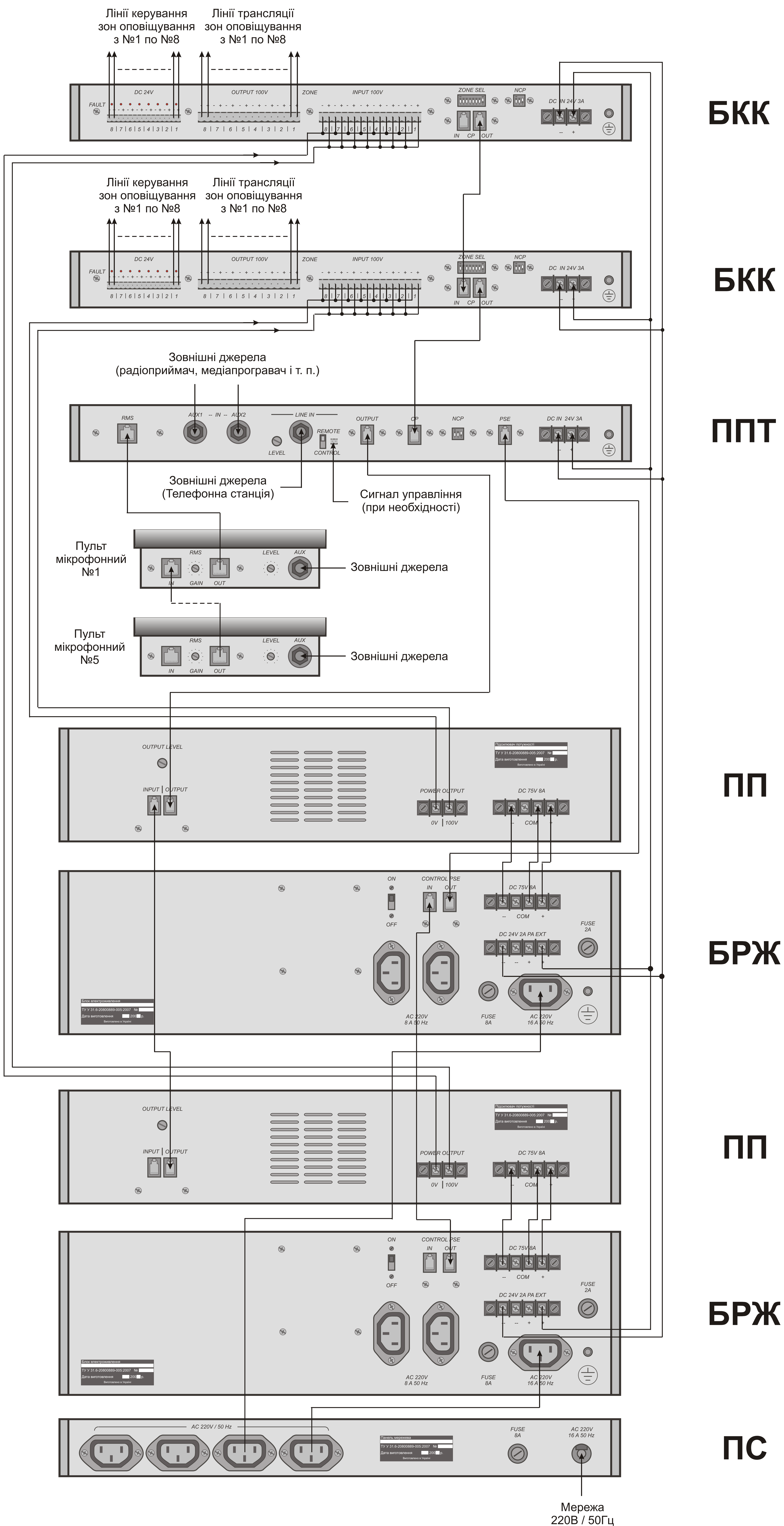
Схема з'єднань елементів устаткування з резервуванням живлення
