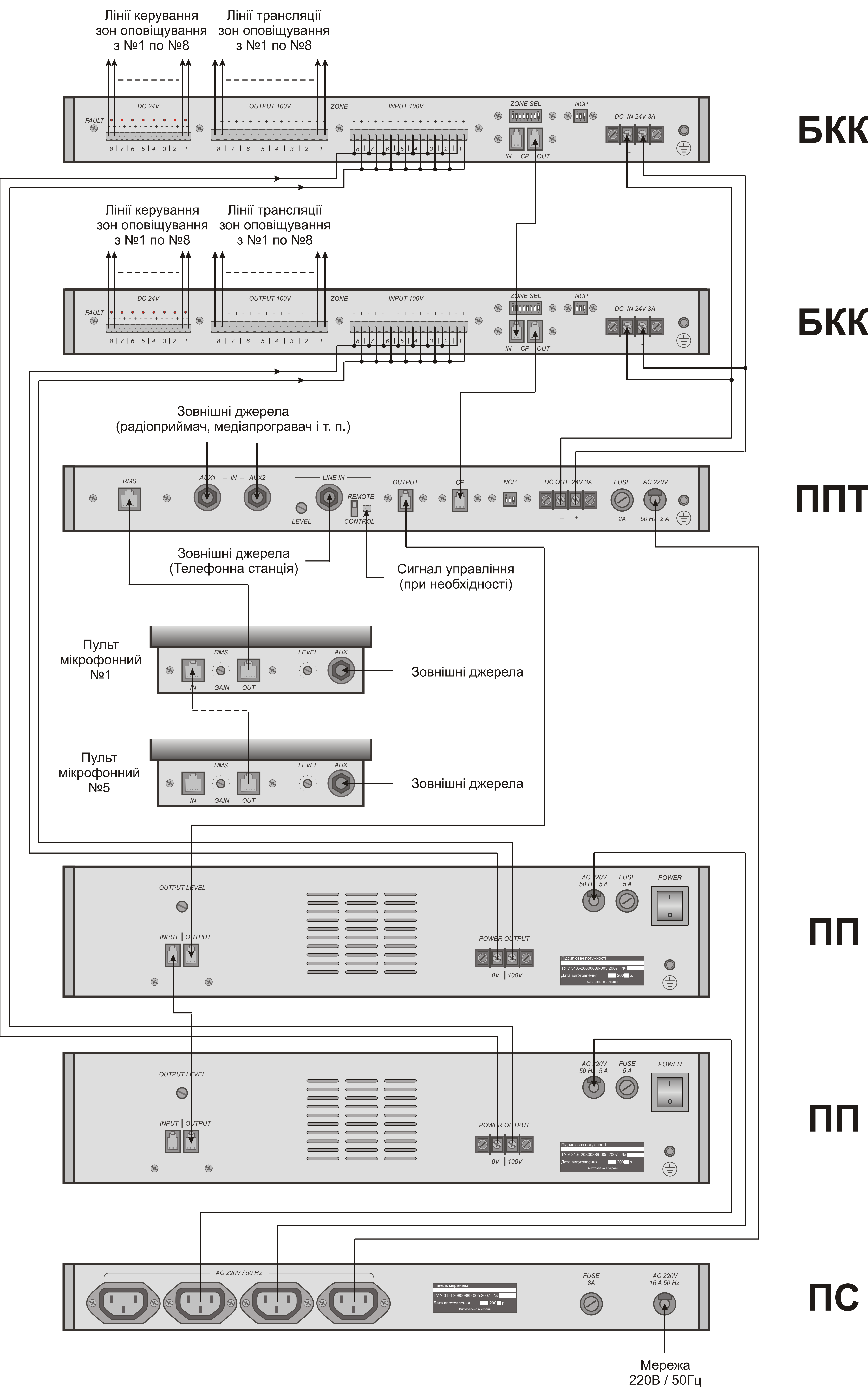
Схема з'єднань елементів устаткування без резервного живлення
