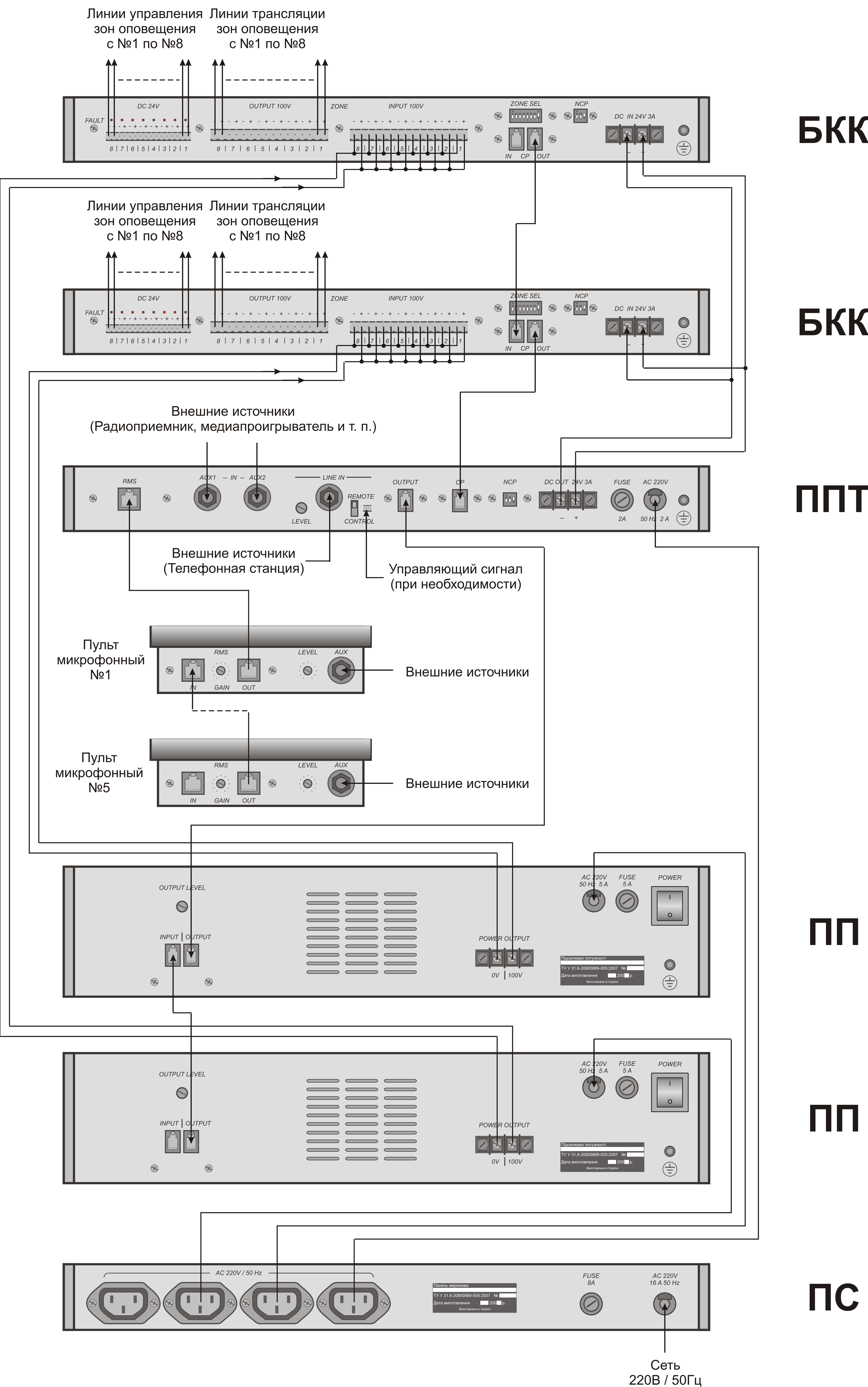
Схема соединений компонентов оборудования без резервного питания
