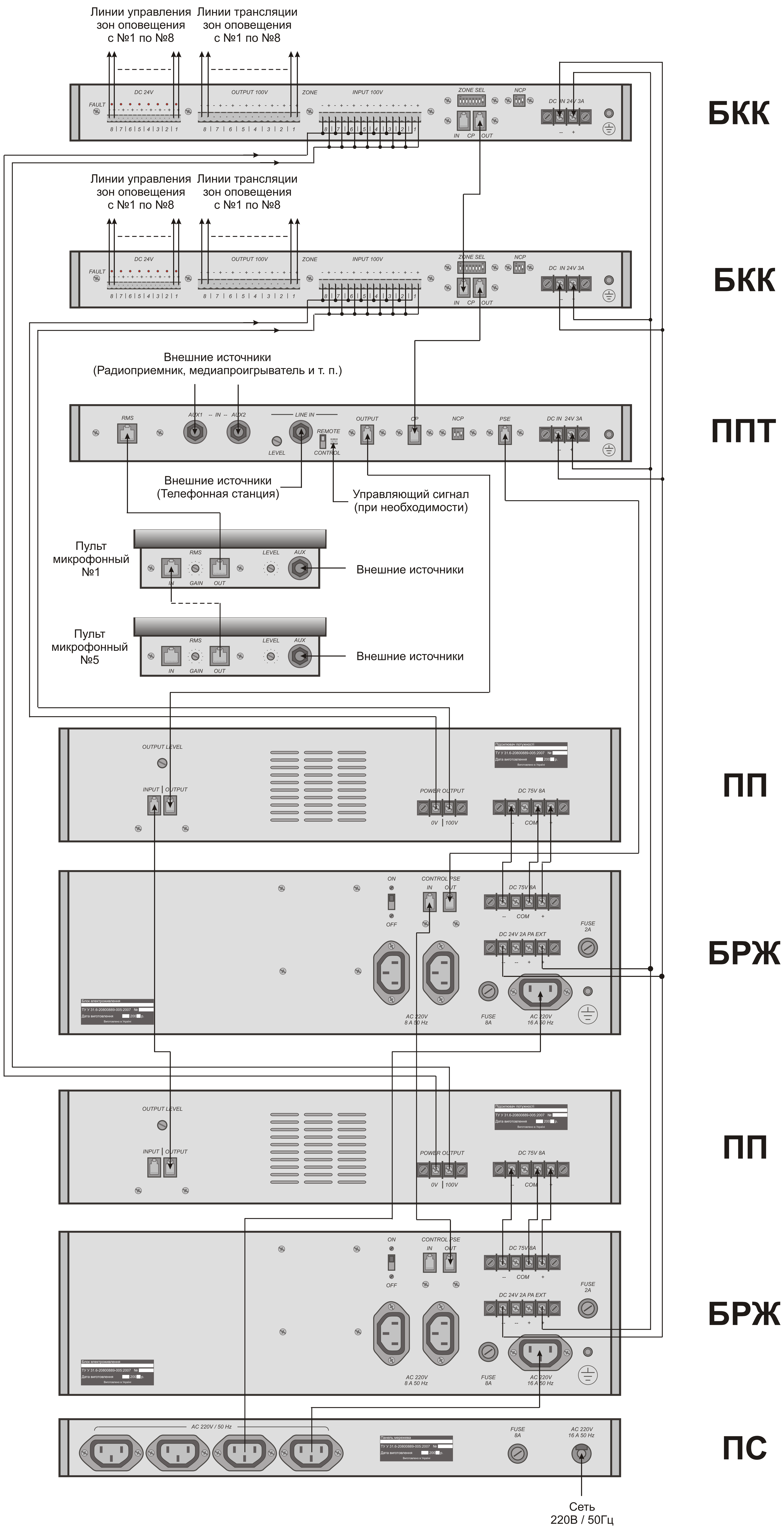
Схема соединений компонентов оборудования с резервированием питания
