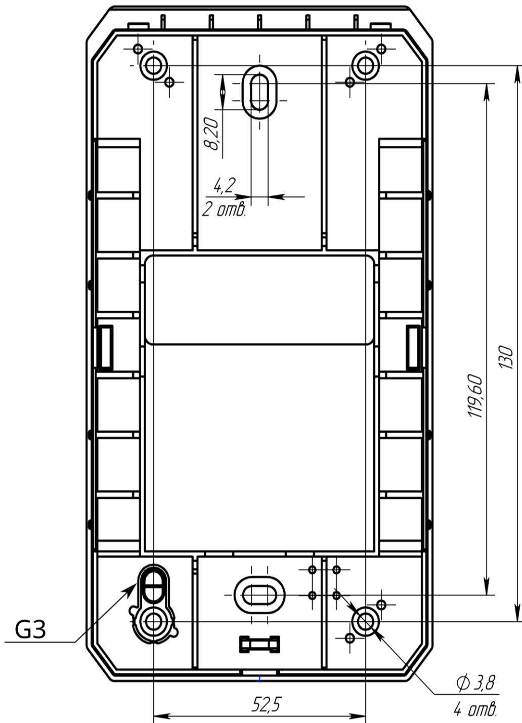
Рисунок 1 – Установчі розміри клавіатури
