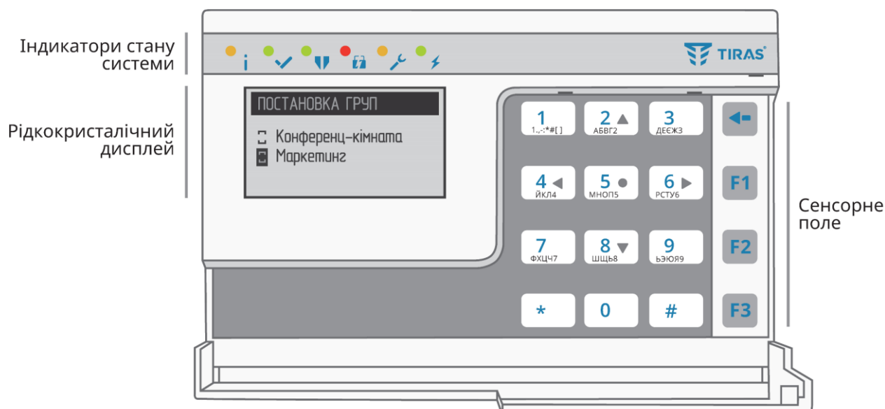
Рисунок 2.1 – Клавіатура K-LCD
