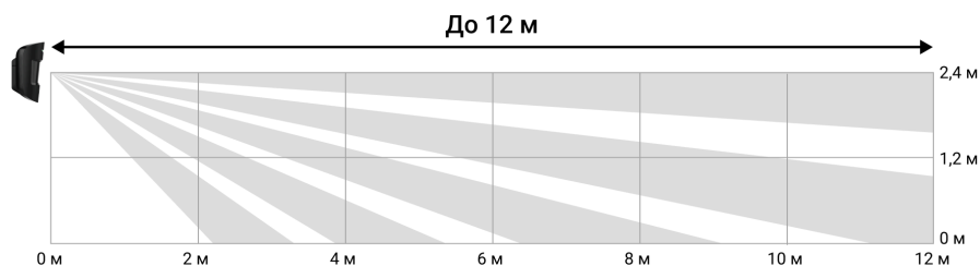
Вертикальний кут огляду датчика
