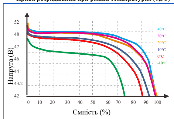
Крива розрядження при різних температурах (0,5C)
