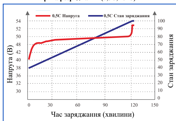
Крива розрядження (0,5C, 25°C)
