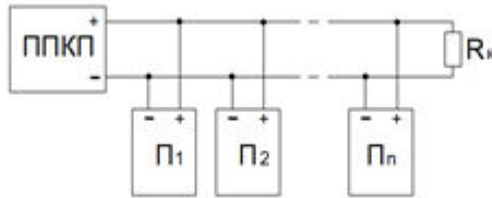
Малюнок 6 Схема живлення показників від ППКП (Прилад приймально- контрольний) R к – кінцевий резистор, номинал визначається ППКП П 1 , П 2 , ... П n – показники з живленням 12 / 24В
