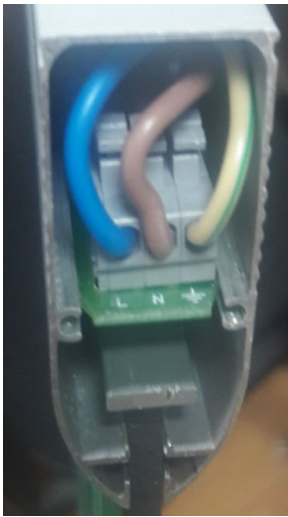
Малюнок 1 Приєднання живлення 230 В
