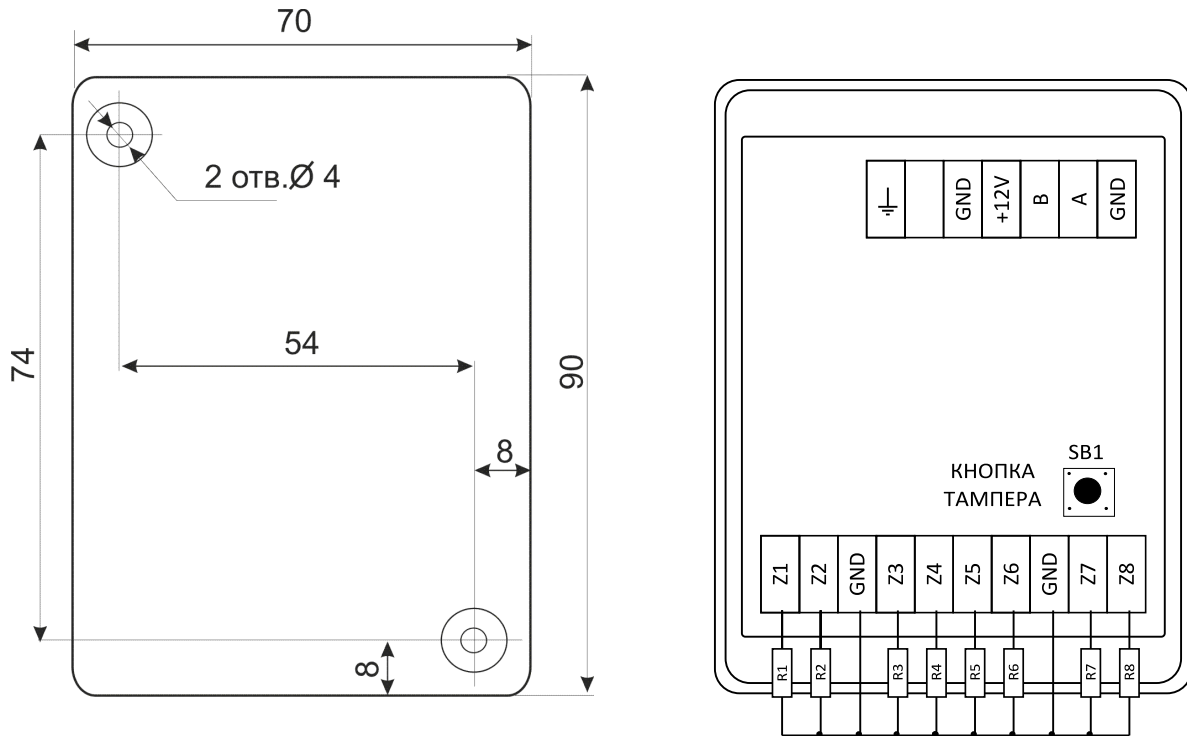
Рисунок 1 – Зовнішній вигляд модуля
