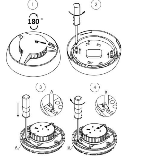
Рисунок 3 – Послідовність кроків для видалення ламкого елемента
