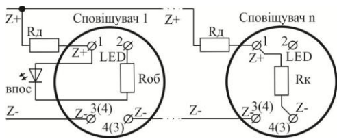
Рисунок 4 – Підключення ВПОС або світлодіода
