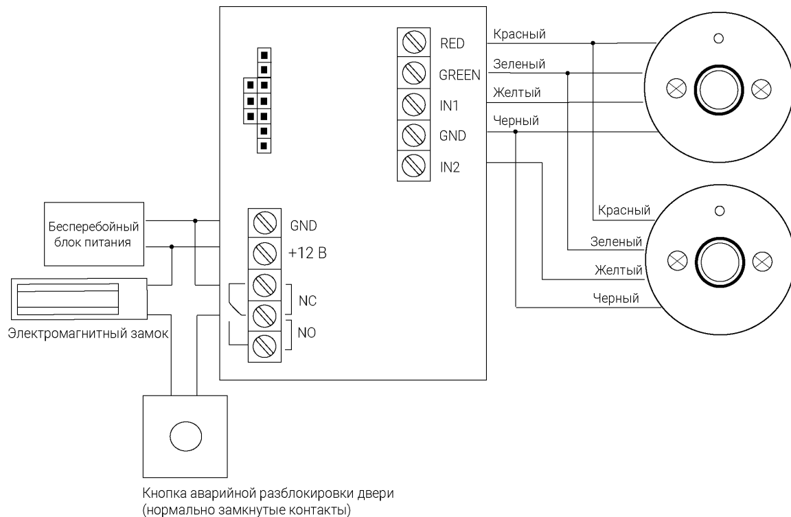
Схема 6 - Подключение контроллера с двумя считывателями Proximity (PR-XX вход и выход) и кнопкой аварийной разблокировки двери
