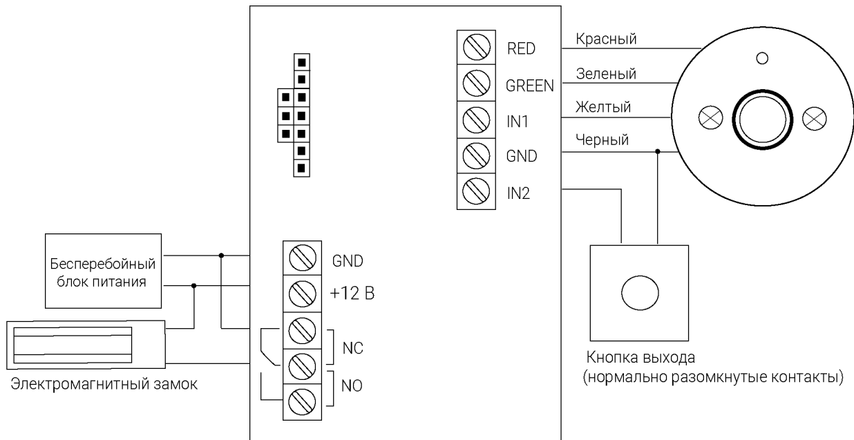
Схема 3 - Подключение контроллера со считывателем Touch Memory (iBR-XX) на вход и кнопкой на выход
