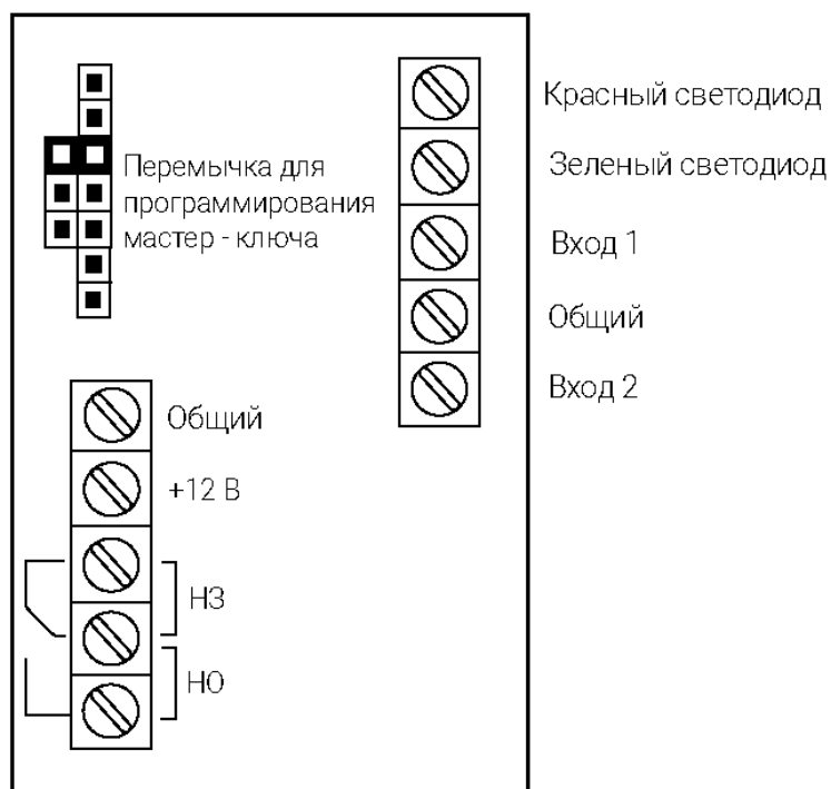
Рисунок 1 – Обозначение разъемов локального модуля контроля доступа iBC - 04
