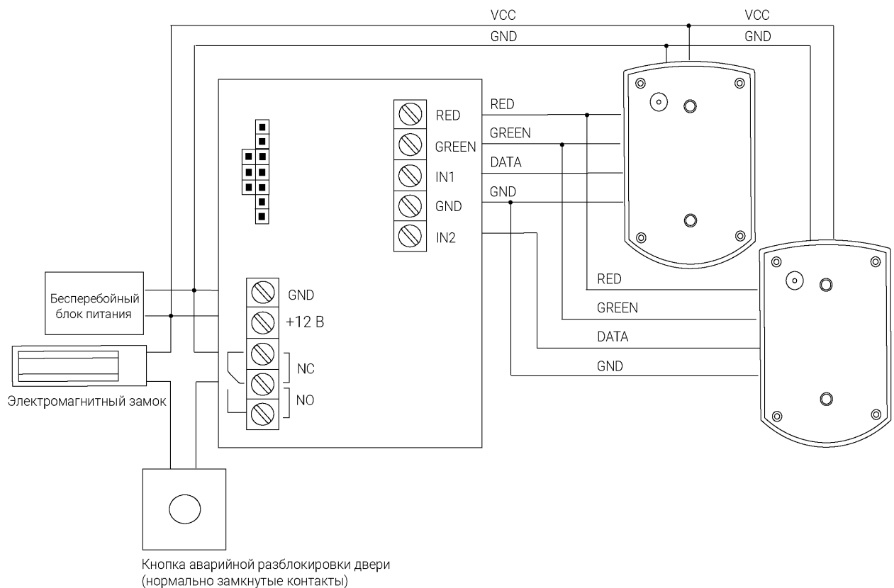
Схема 6 - Подключение контроллера с двумя считывателями Proximity (PR-XX вход и выход) и кнопкой аварийной разблокировки двери
