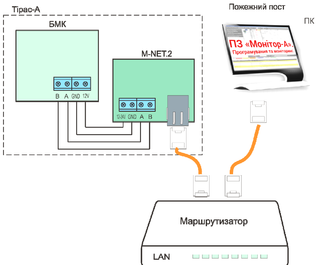
Рисунок 5.7 – Підключення Тірас-А до «Монитор-А» через мережевий маршрутизатор
