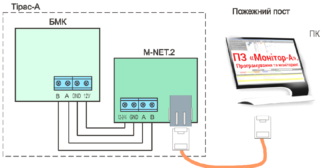
Рисунок 5.6 – Пряме підключення Тірас-А до «Монитор-А»
