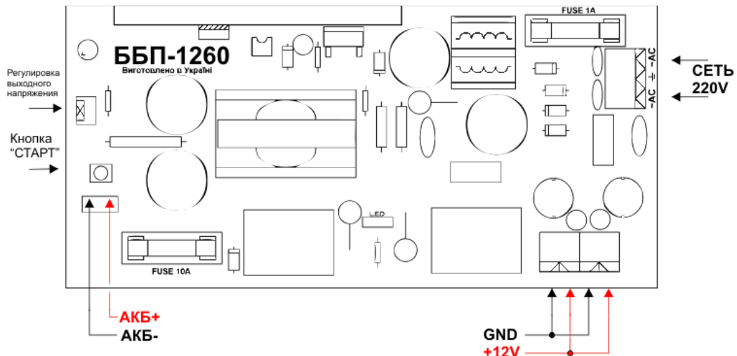
Рис. 2 Схема подключения блок питания
