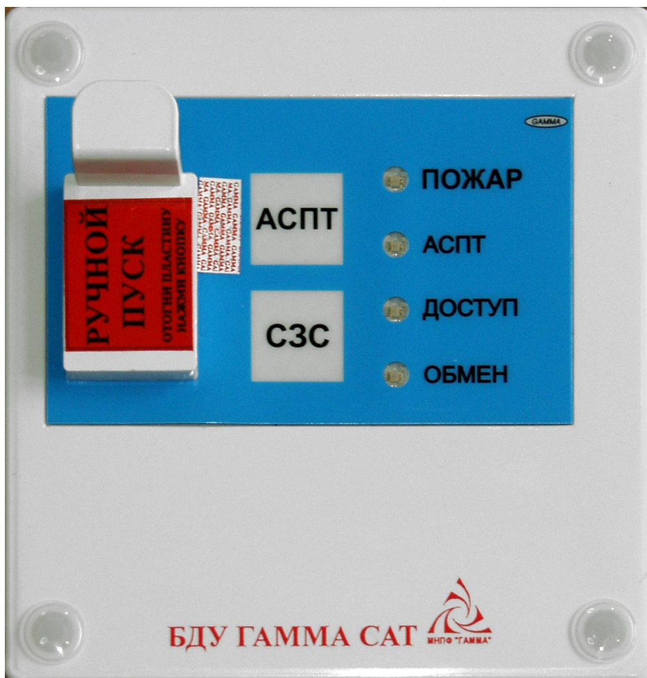
Рисунок 1. Общий вид БДУ предыдущей модификации
