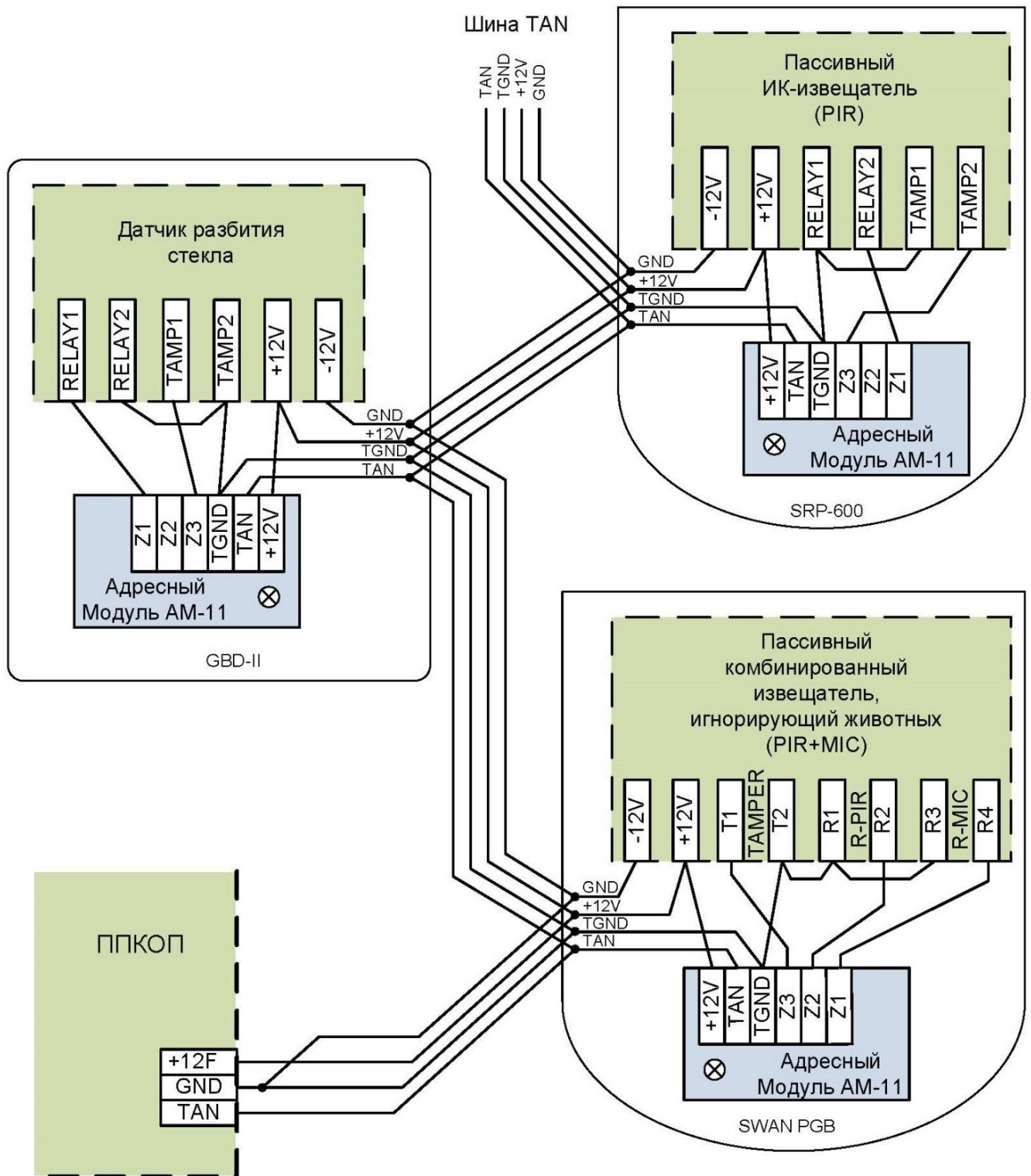
Рисунок 27. Пример использования адресных модулей «AM-11»
