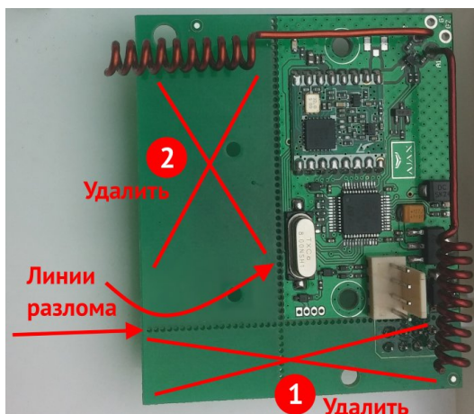
Рисунок 20. Подготовка радиоприемника Ajax «uartBridge»
