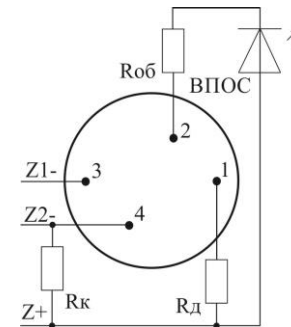
Рисунок 3 – Підключення ВПОС або світлодіода
