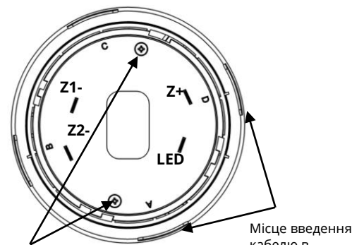
Кріплення верхньої кришки сповіщувача Рисунок 2 – Вигляд сповіщувача з боку контактів
