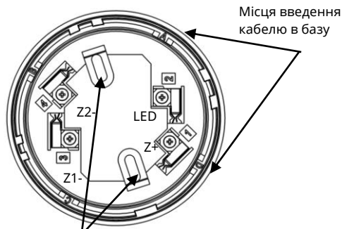
Місця кріплення бази до поверхні Рисунок 1 – Розташування клем на базі сповіщувача
