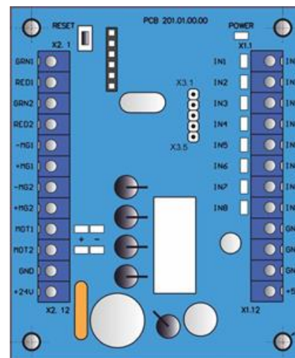
Рис. 9 – Зовнішній вигляд контролера моторизованого механізму PCB.201.01.00.00
