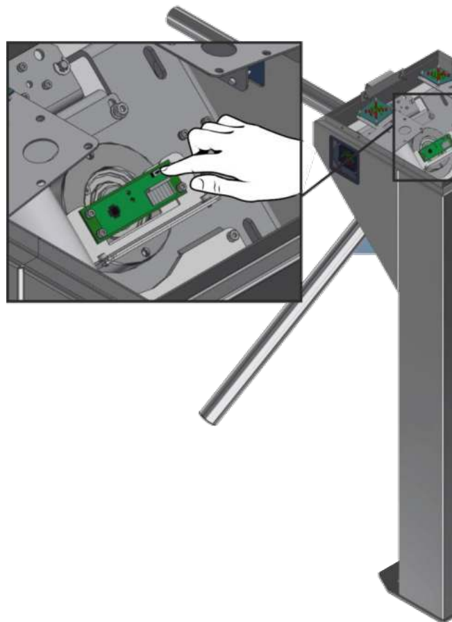
Рис. 18 – Встановлення нульового положення ступиці
