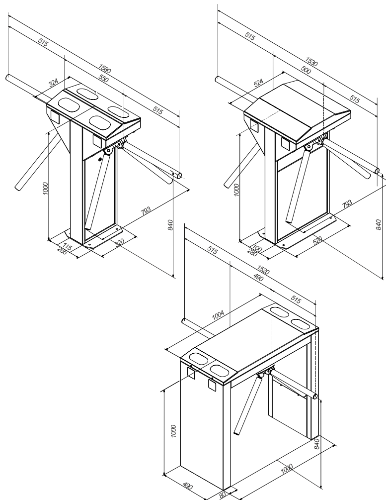
Рис. 3 - Габаритні розміри турнікету-триподу
