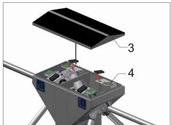
Рис. 17– Встановлення зчитувача в турнікет-трипод
