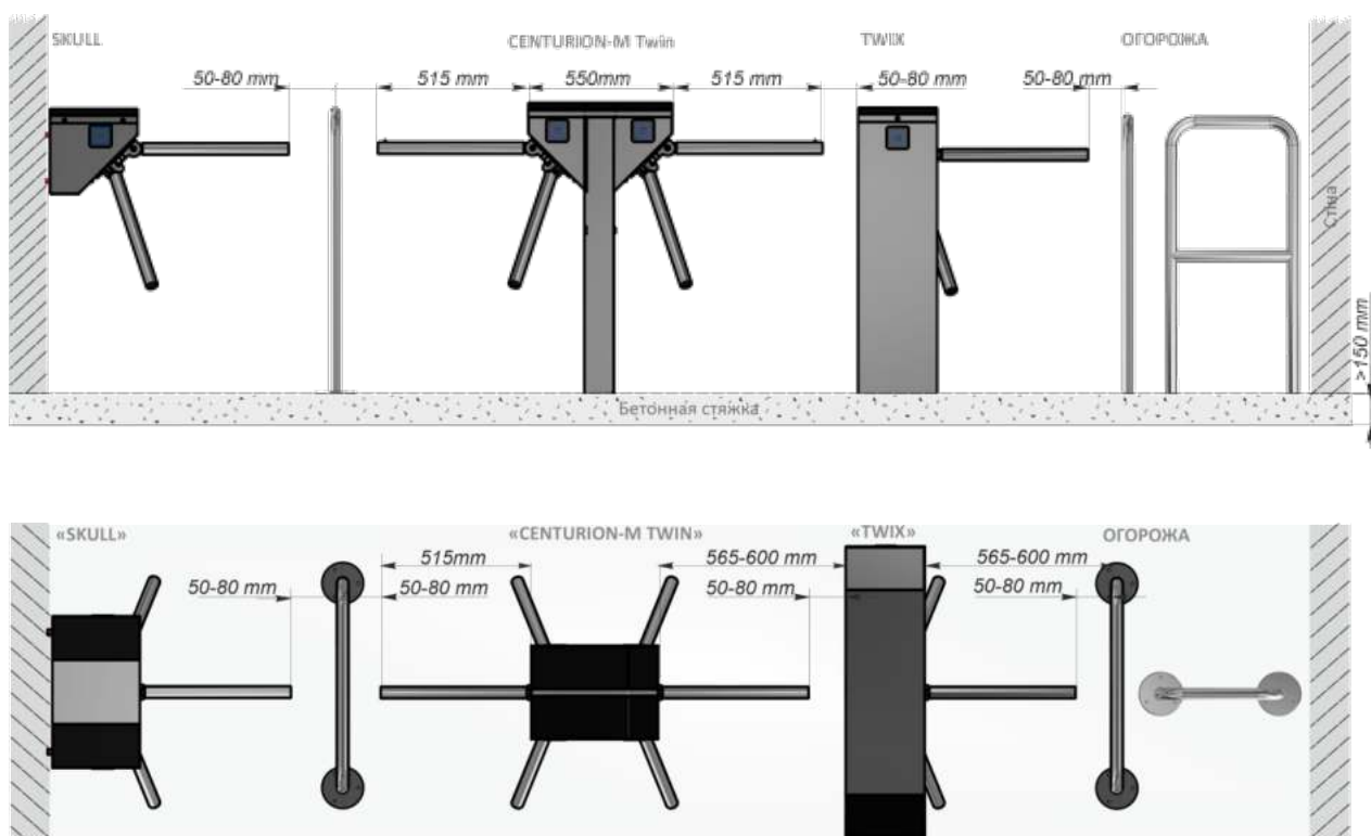
Рис.12 –Інсталяція розміщення турнікетів-триподів одно- та двосторонніх (умовно)
