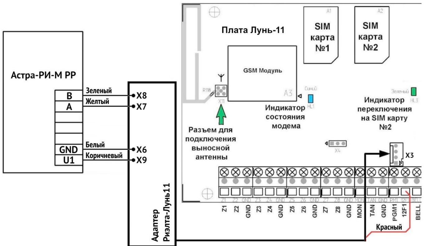
Рисунок 44. Схема подключения РПУ «Астра RI-M PP»
