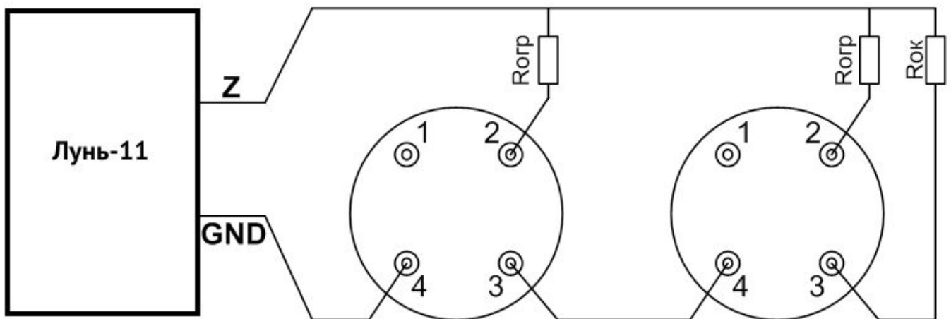
Рисунок 38. Схема подключения извещателей в пожарный шлейф по двухпроводной схеме
