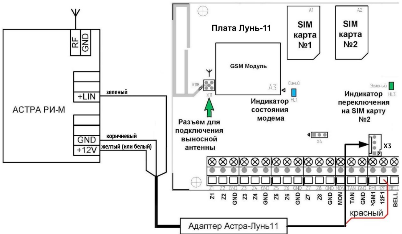
Рисунок 43. Схема подключения РПУ «Астра RI-M»
