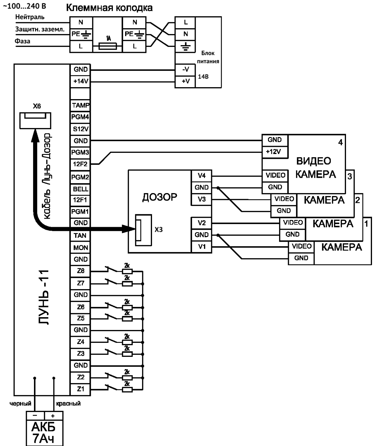
Рисунок 42. Схема подключения модуля фотоподтверждения тревог «Дозор»
