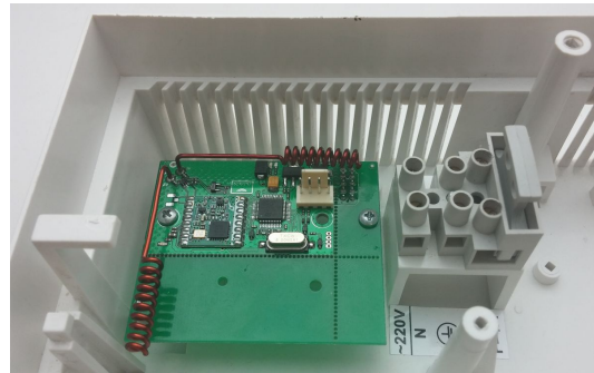
Рисунок 29. Радиоприемник Ajax «uartBridge» в корпусе прибора
