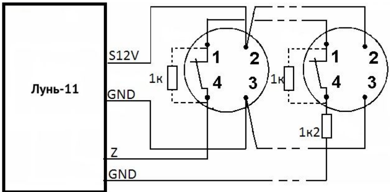
Рисунок 37. Схема подключения пожарных извещателей по четырехпроводной схеме
