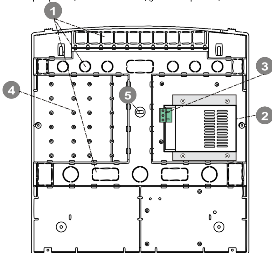
Рисунок 3 – Зовнішній вигляд корпусу без основного модуля «Tiras PRIME 4/8/16»:
