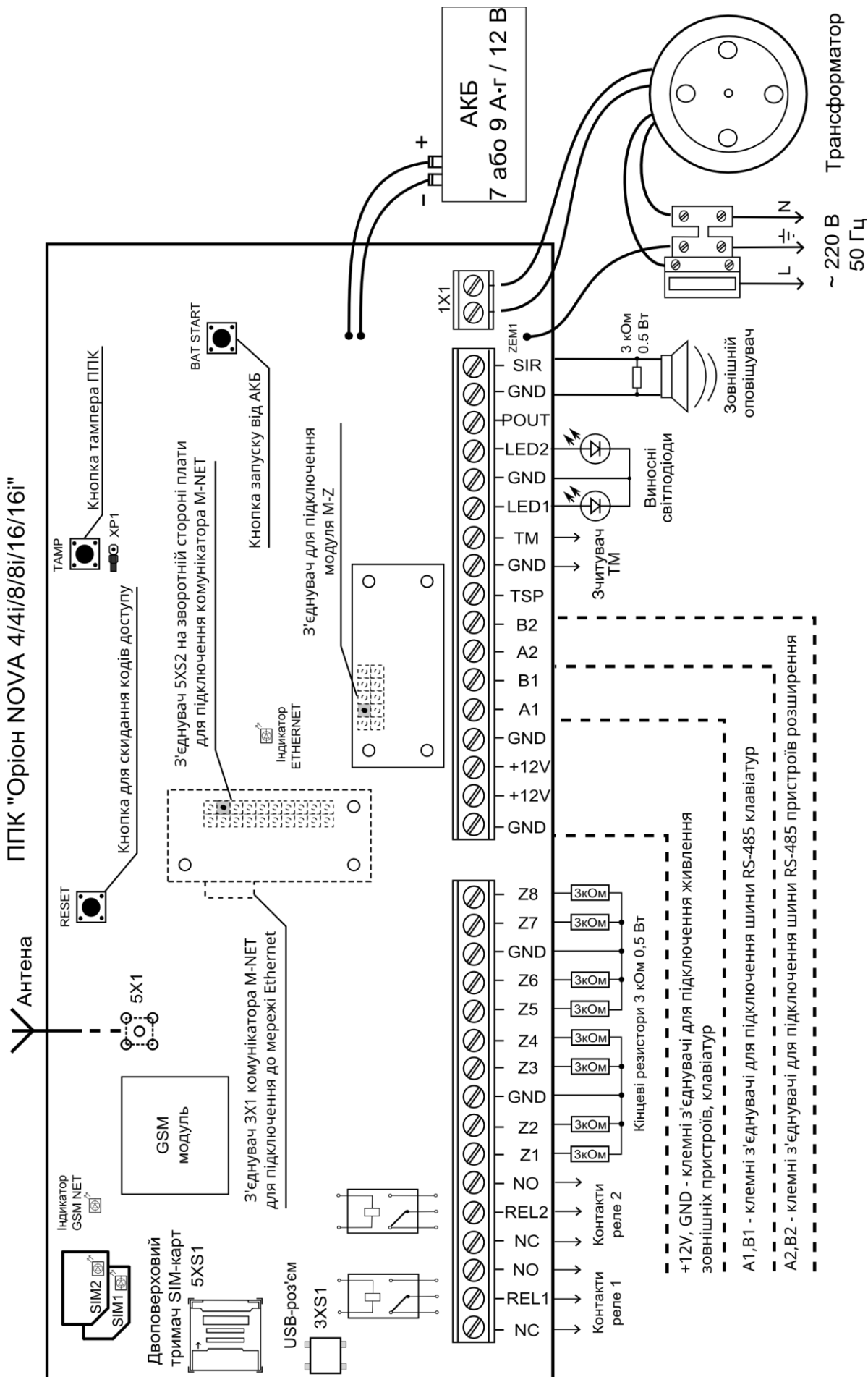
Рисунок Б.1 - Схема електрична підключення ППК
