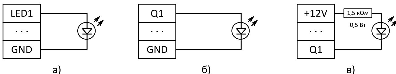
а) – до ППК або М-ZP box, б) – до клавіатури (виносний світлодіод), в) – до клавіатури (відкритий колектор)
