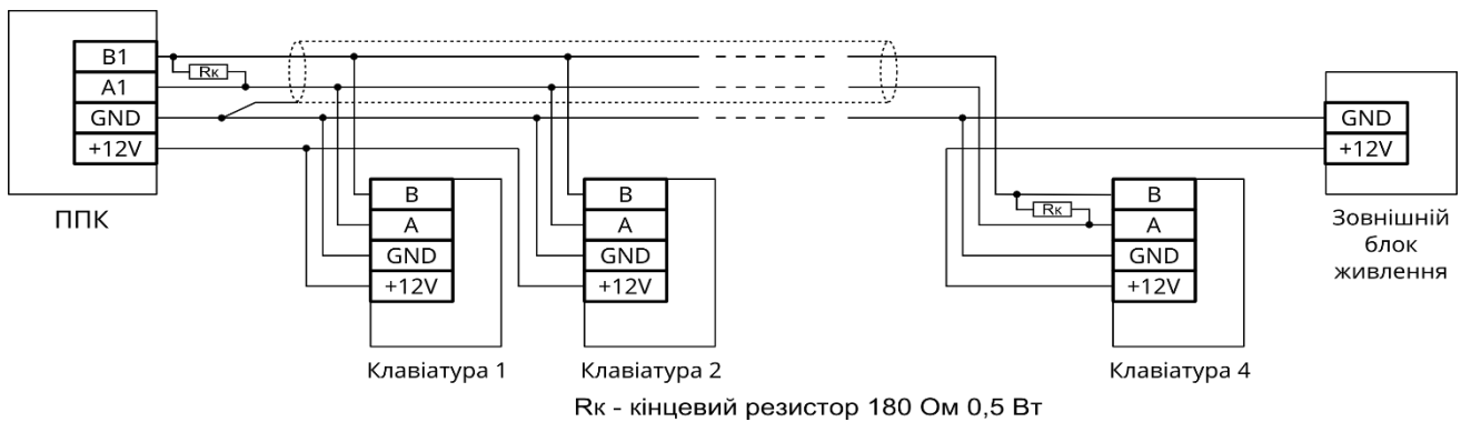
Рисунок 2.2 – Приклад підключення клавіатур по шині RS-485
