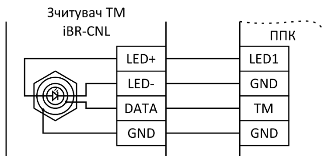
Рисунок 2.6 – Схема підключення зчитувача ключів Touch Memory
