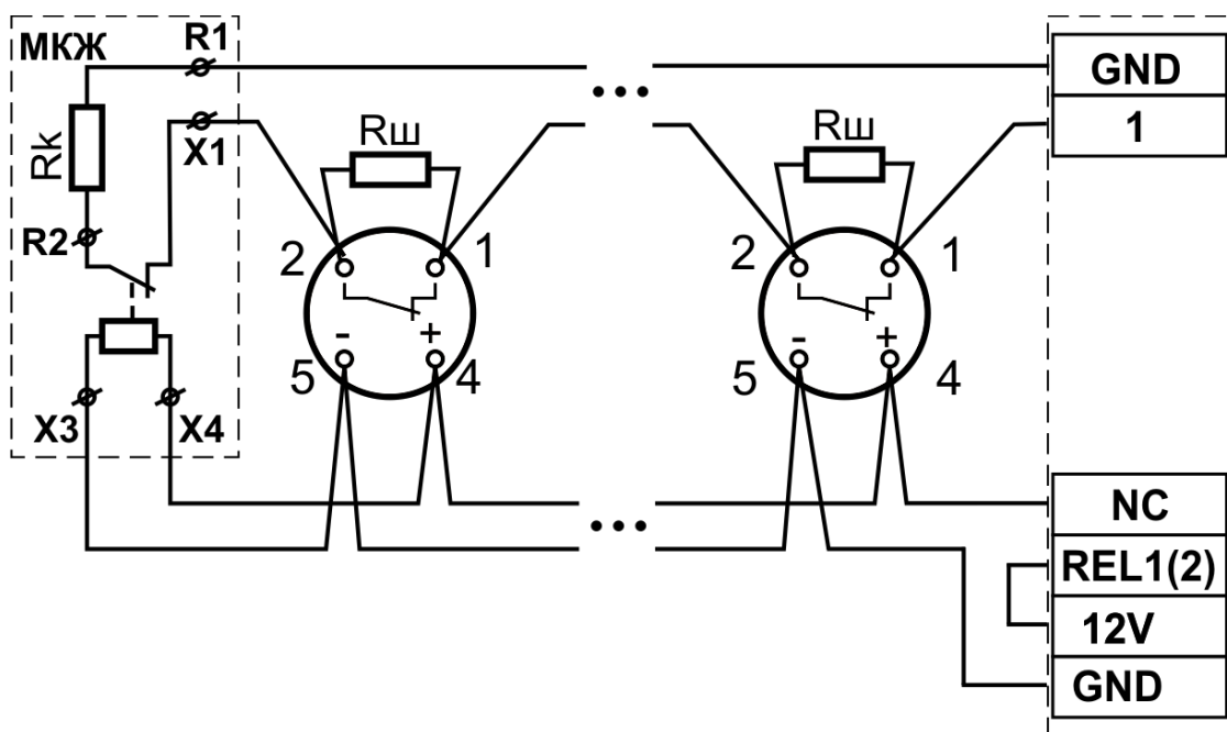
Рисунок 7.2 – Приклад підключення чотирипровідних сповіщувачів з живленням від приладу.
