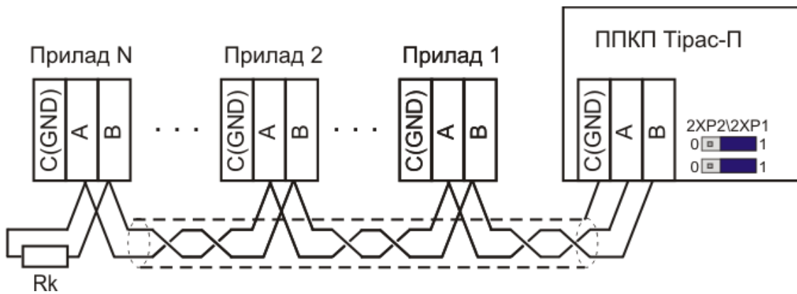
Рисунок 7.5- Підключення інтерфейсу RS-485 без відгалужень
