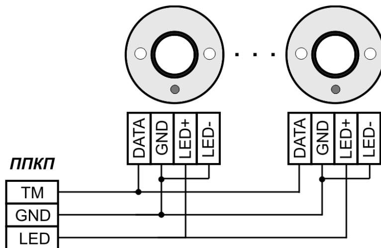
Рисунок 7.4 – Підключення Touch Memory
