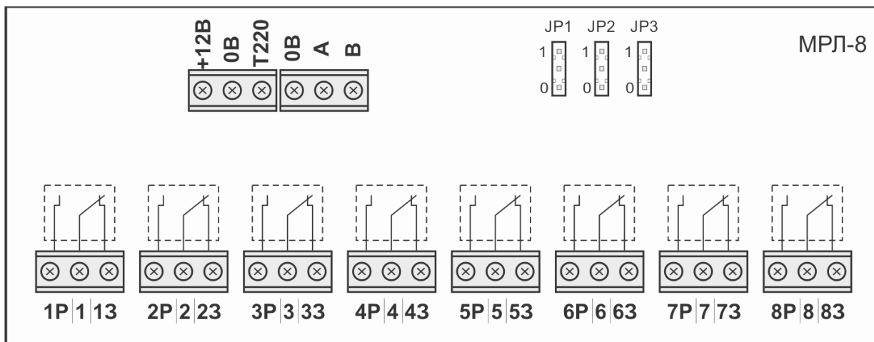
Рисунок 7.9 – Підключення входів та виходів МРЛ-8
