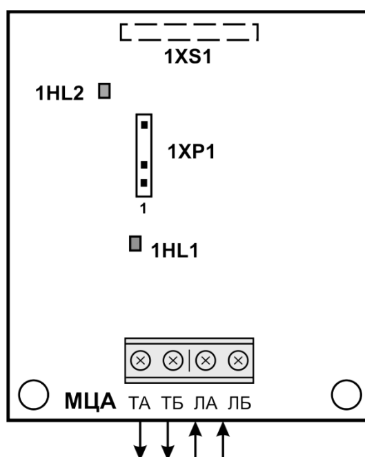
Рисунок 7.10 – Підключення входів та виходів МЦА
