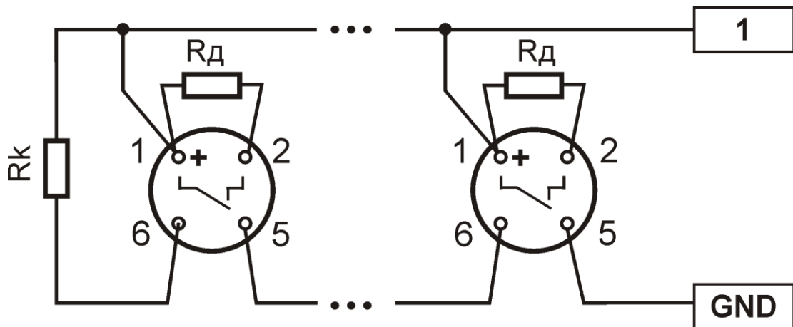
Рисунок 7.1 – Підключення двопрвідних сповіщувачів
