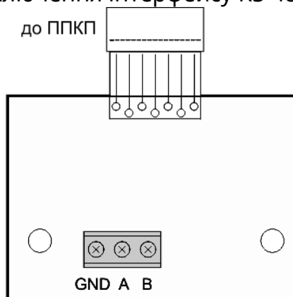
Рисунок 7.5- Підключення інтерфейсу RS-485 без відгалужень
