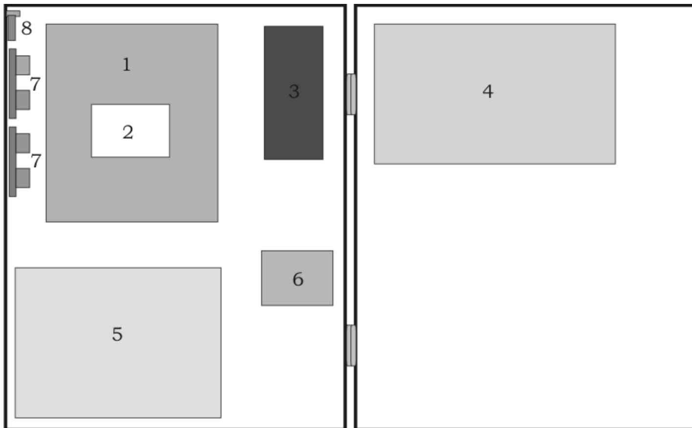
Рисунок Б.1 – Розміщення блоків та модулів в корпусі приладу
