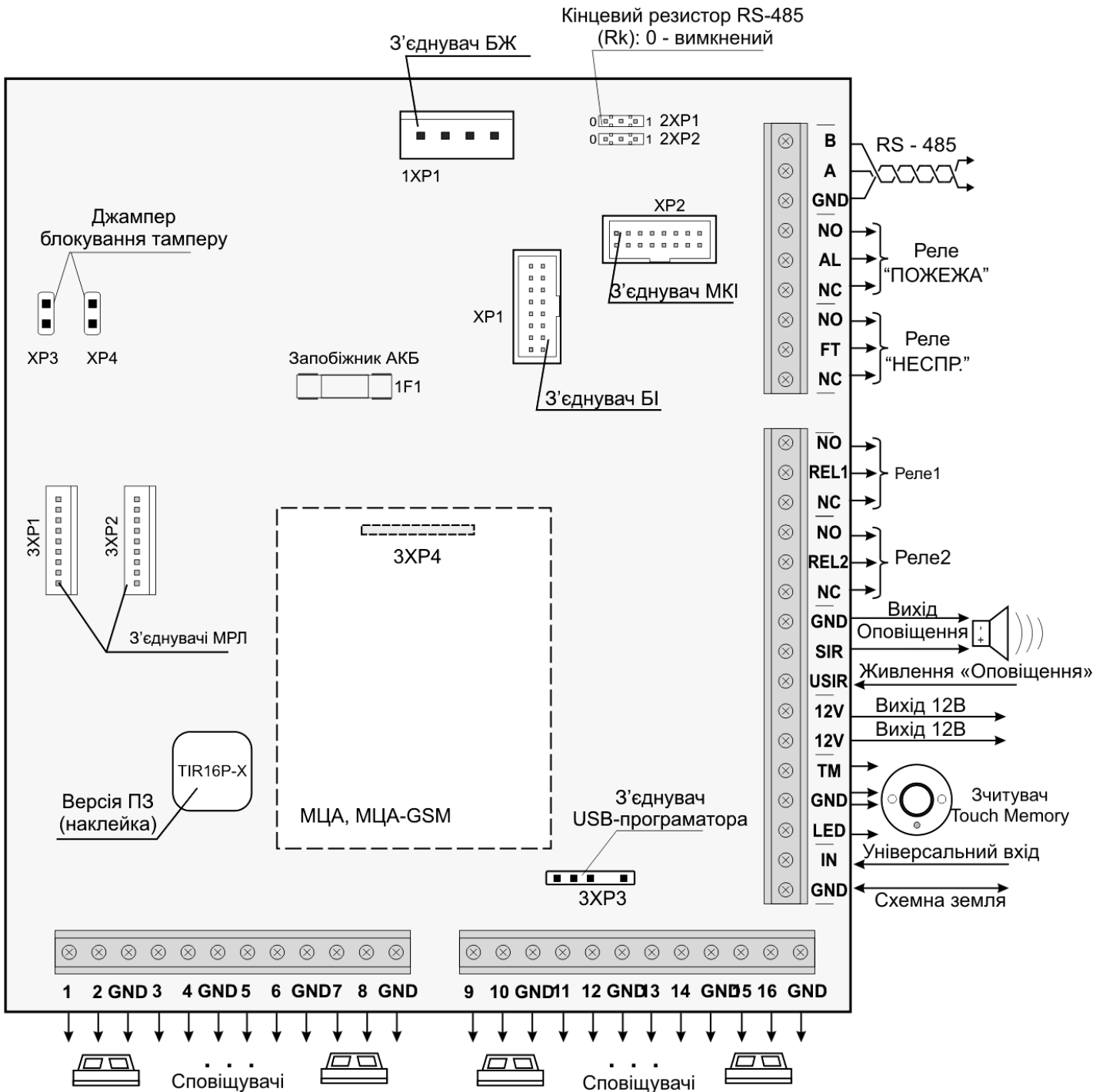
Рисунок Г.1 – Схема електричних з'єднань.
