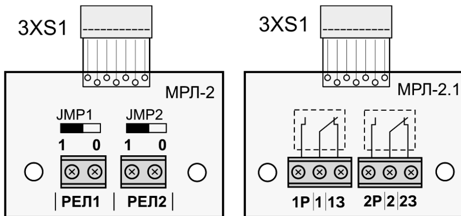
Рисунок 7.8 – Модулі МРЛ
