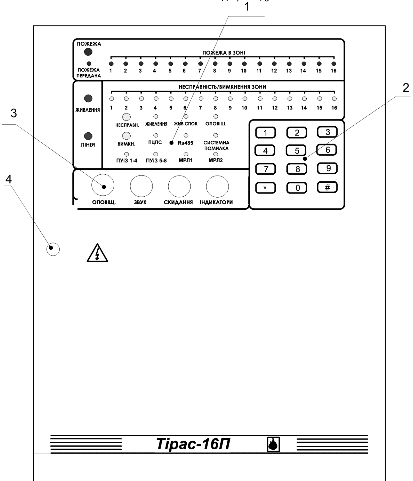
Рисунок А.1 – Зовнішній вигляд приладу
