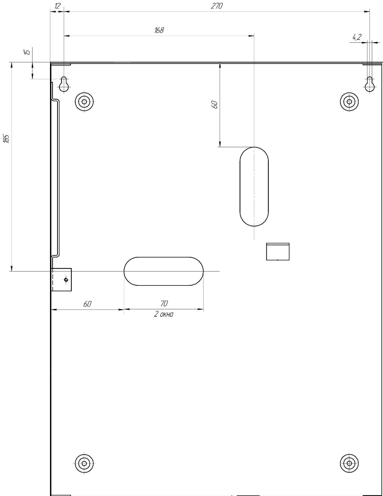
Рисунок В.1 – Розмітка отворів кріплення приладу
