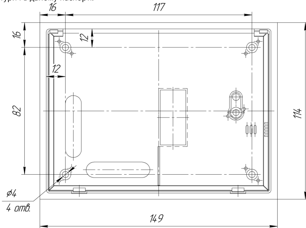
Рисунок 1 – Установчі розміри клавіатури K-GLCD
