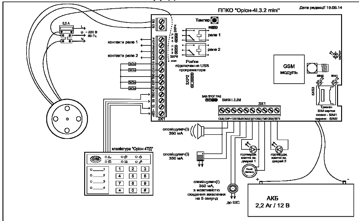
Рисунок А.1 - Схема електрична підключення ППКО «Оріон-4І.3.2 mini»
