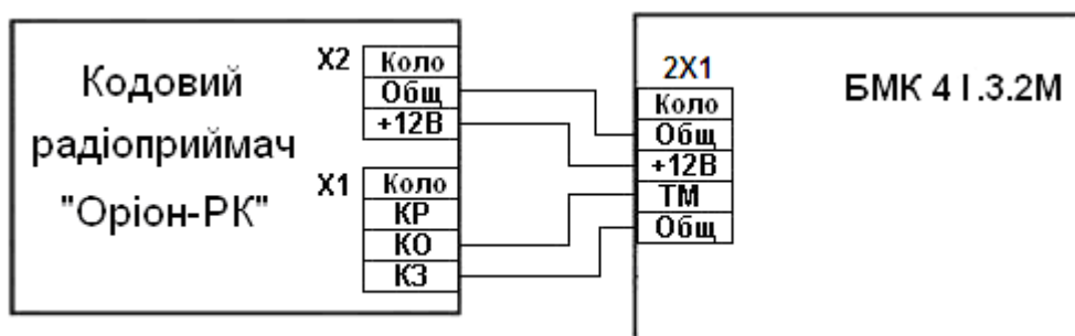
Рисунок 3 - Схема підключення кодового радіоприймача «Оріон-РК»
