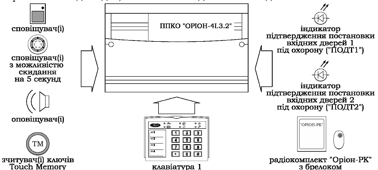
Рисунок 1 – ППКО «Оріон-4І.3.2» в повному складі
