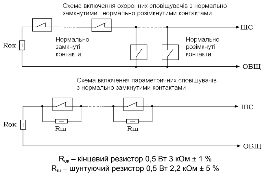
Рисунок 3 – Схеми включення сповіщувачів
