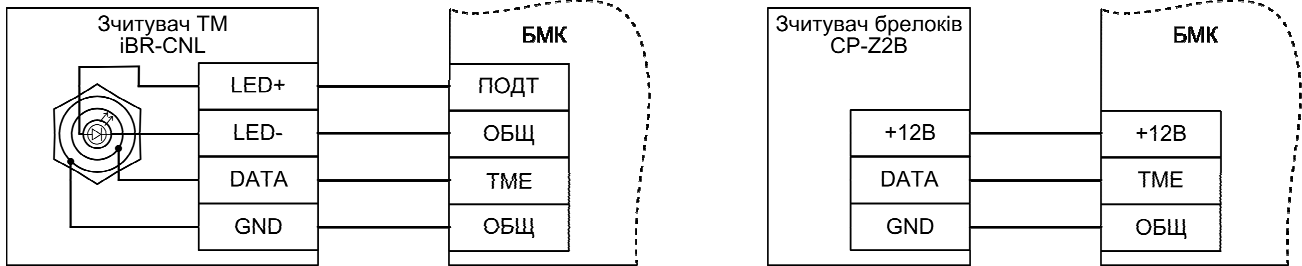
Рисунок 4 - Схема підключення зчитувача ключів ТМ (ліворуч) та зчитувача Proximity брелоків (праворуч)
