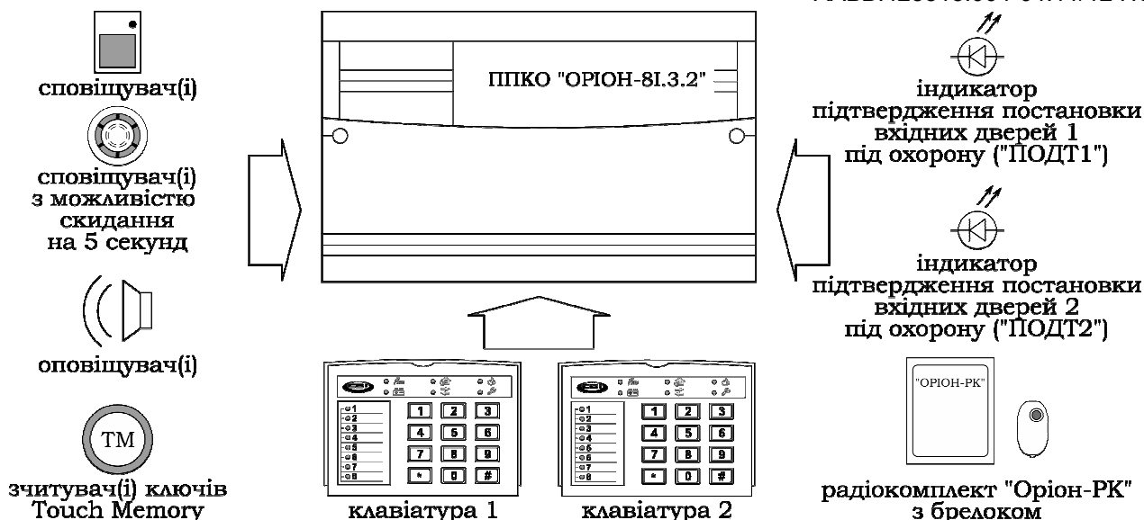
Рисунок 2 – ППКО «Оріон-8І.3.2» в повному складі
