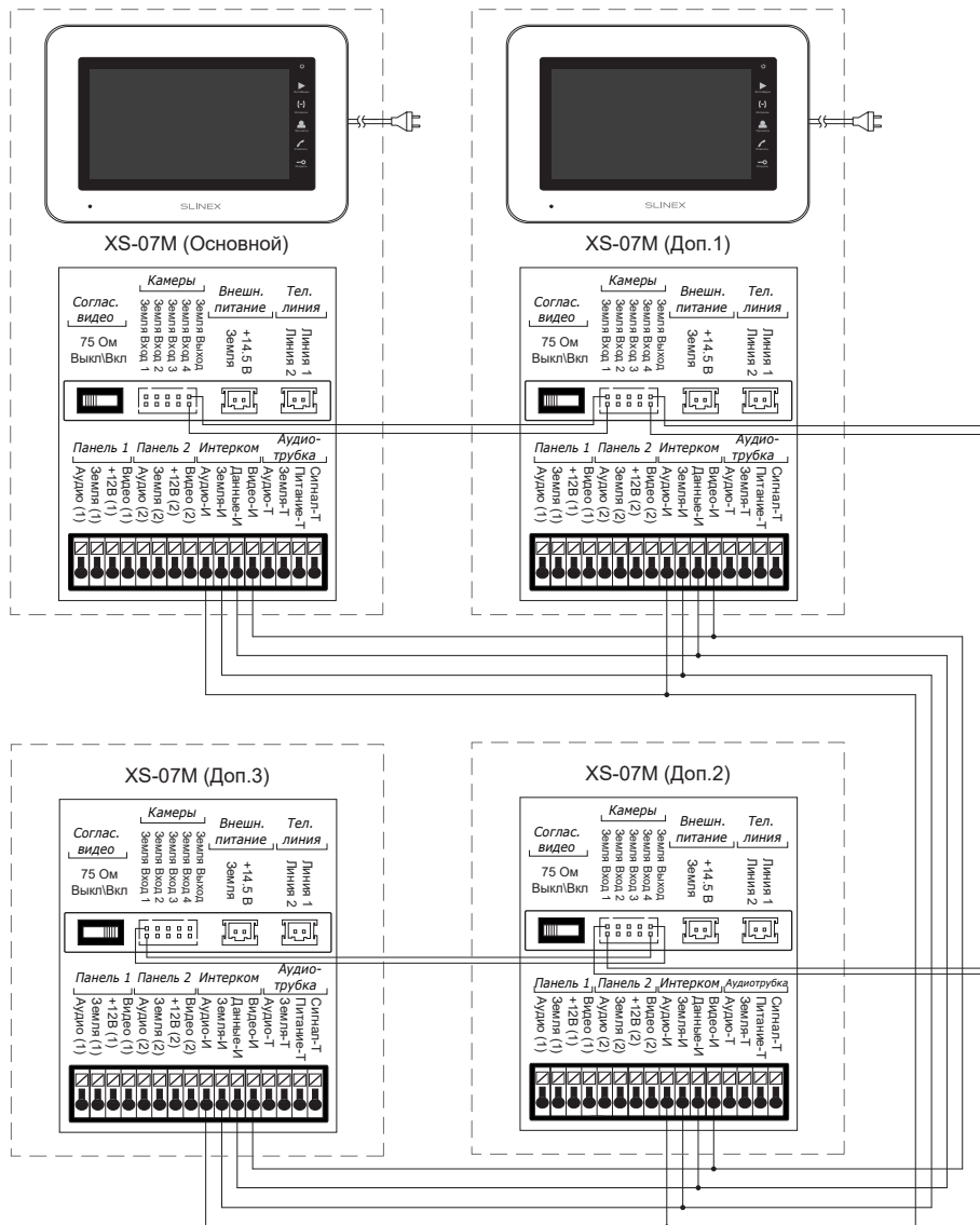
Схема 4. Подключение системы домофонов XS-07М в режиме CCTV2 – камеры подключаются только к «Основному» монитору. При этом просмотр камер возможен с любого монитора в системе.
