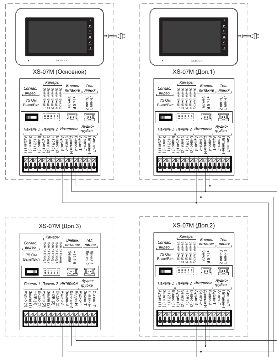
Схема 3. Подключение системы домофонов XS-07M в режиме CCTV – камеры могут быть подключены к любому монитору в системе. При этом просмотр камер возможен только на мониторе, к которому они подключены.
