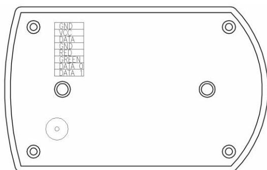
Рис. 1. Подключение по интерфейсу 1-Wire
