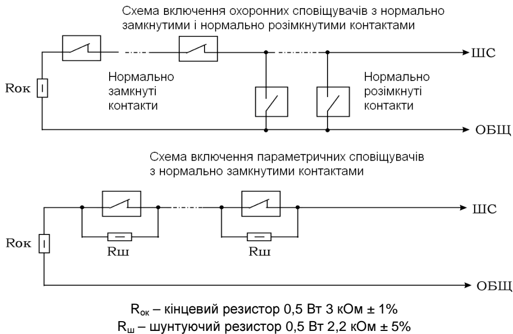
Рисунок 2 – Схеми включення сповіщувачів
