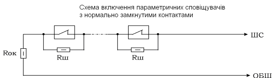
Рисунок 2 – Схеми включення сповіщувачів
