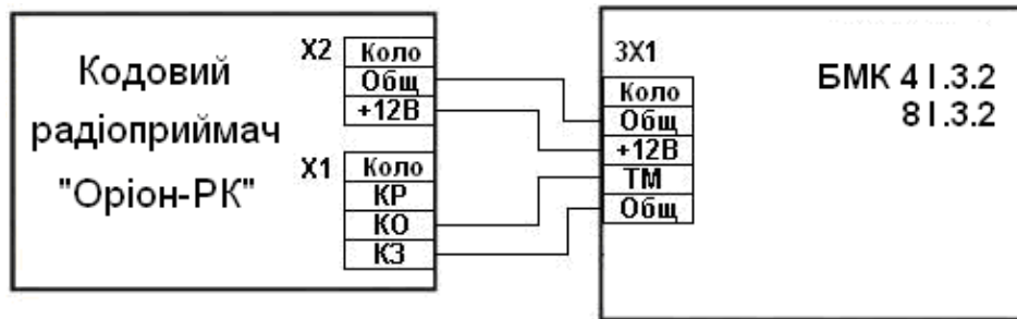
Рисунок 3 - Схема підключення кодового радіоприймача «Оріон-РК»
