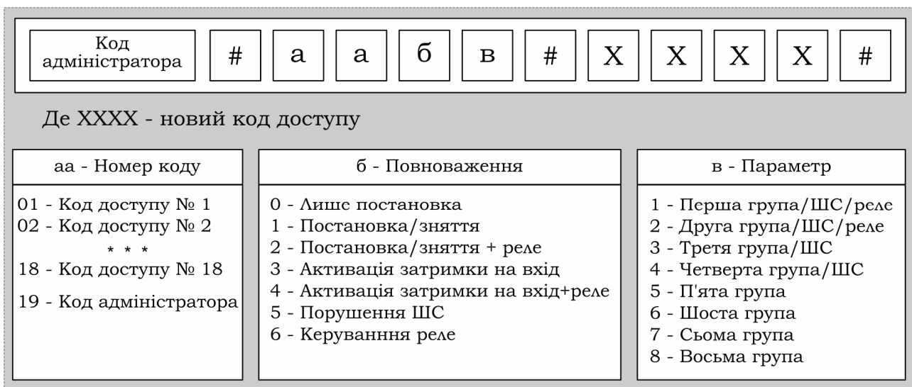
Рисунок 5 – Програмування кодів доступу
