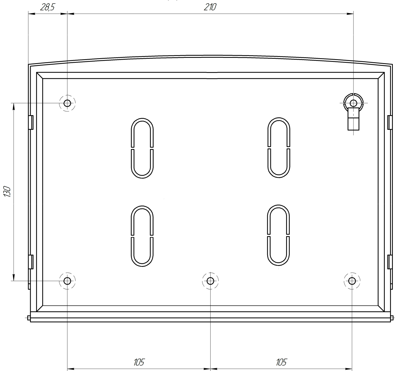
Рисунок В.1 – Установчі розміри ППКО
